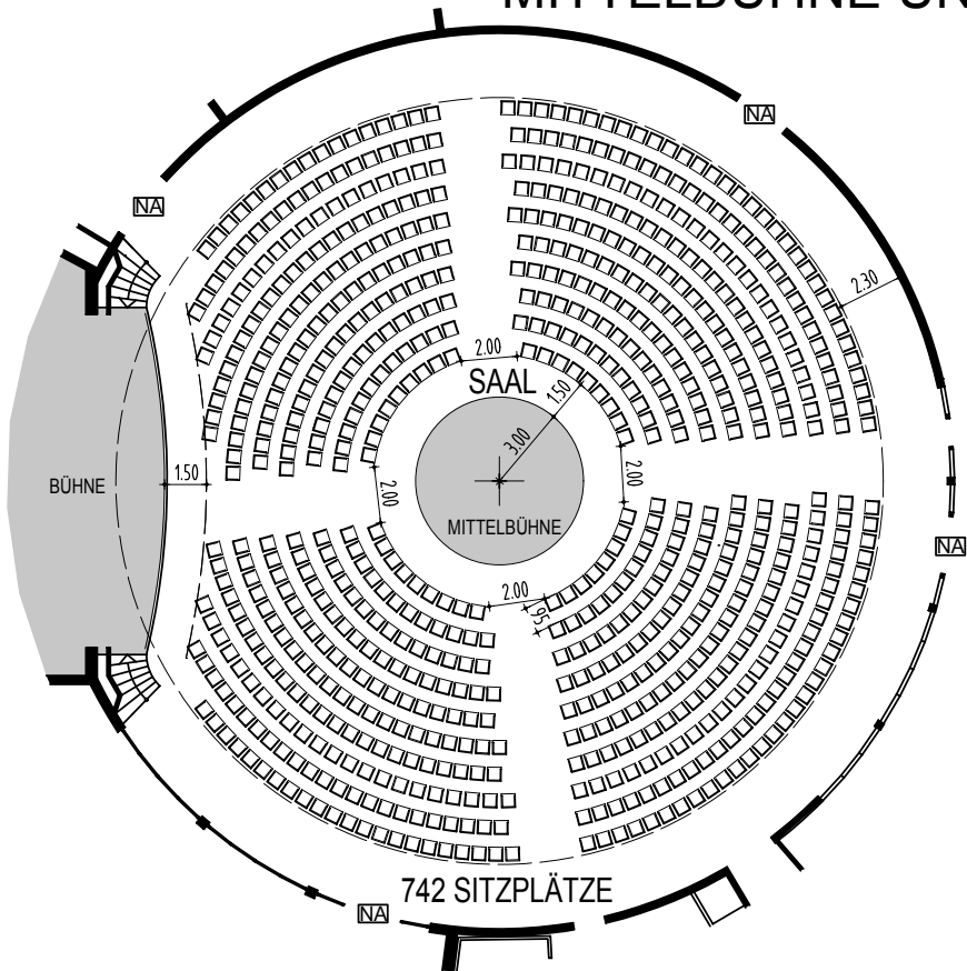
STERNBESTUHLUNG MIT MITTELBÜHNE
